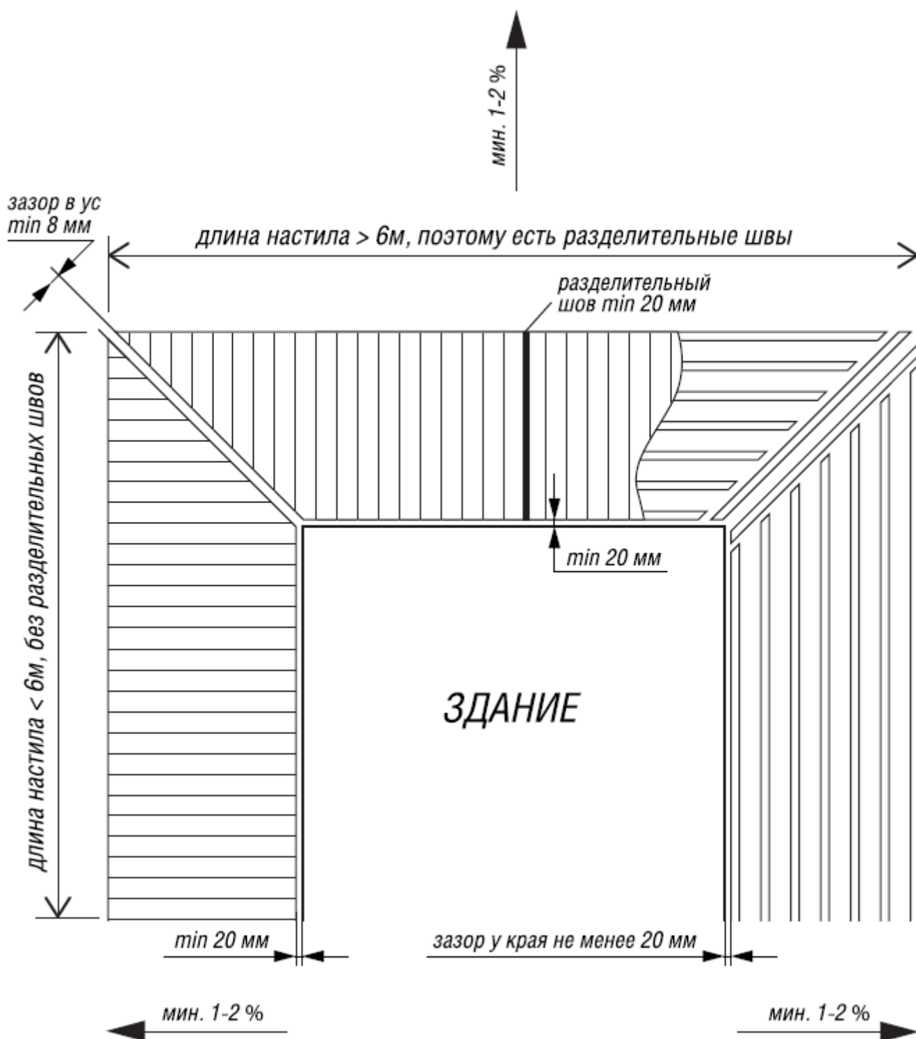
Рис. 17 - Вариант укладки террасного настила вокруг здания Г- или П-образной формы с двумя швами при соединении в ус и одним разделительным швом по ширине настила.
